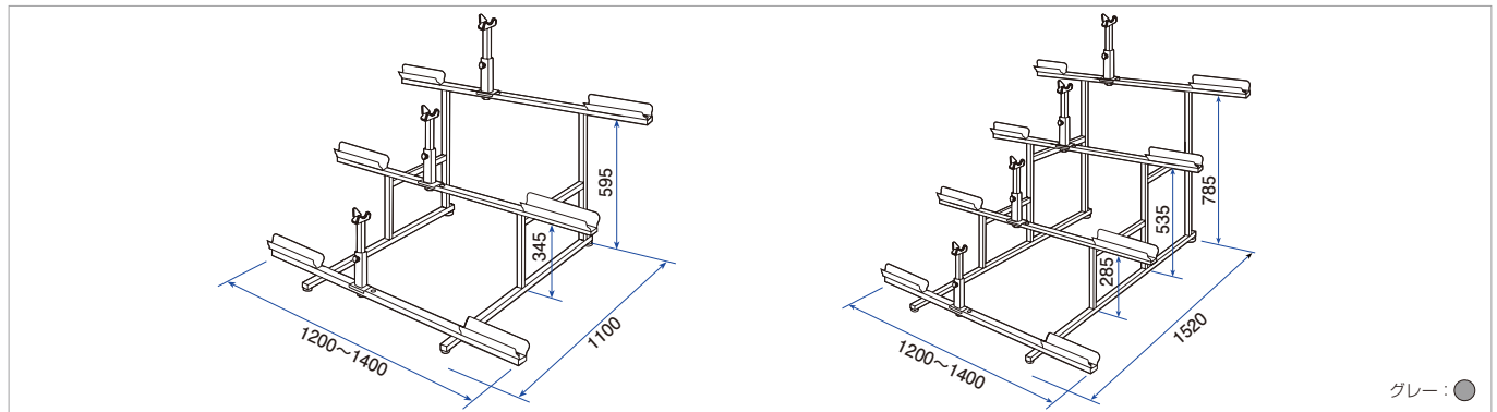
スライド型(3段)
