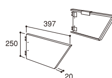
サイドパネルセット
