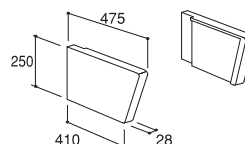
サイドカバーセット<傾斜型>
