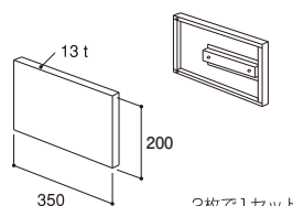
パラペットカバーセット
