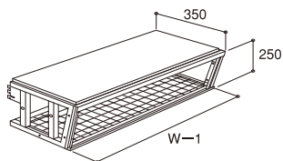
パラペットセット<傾斜型>
